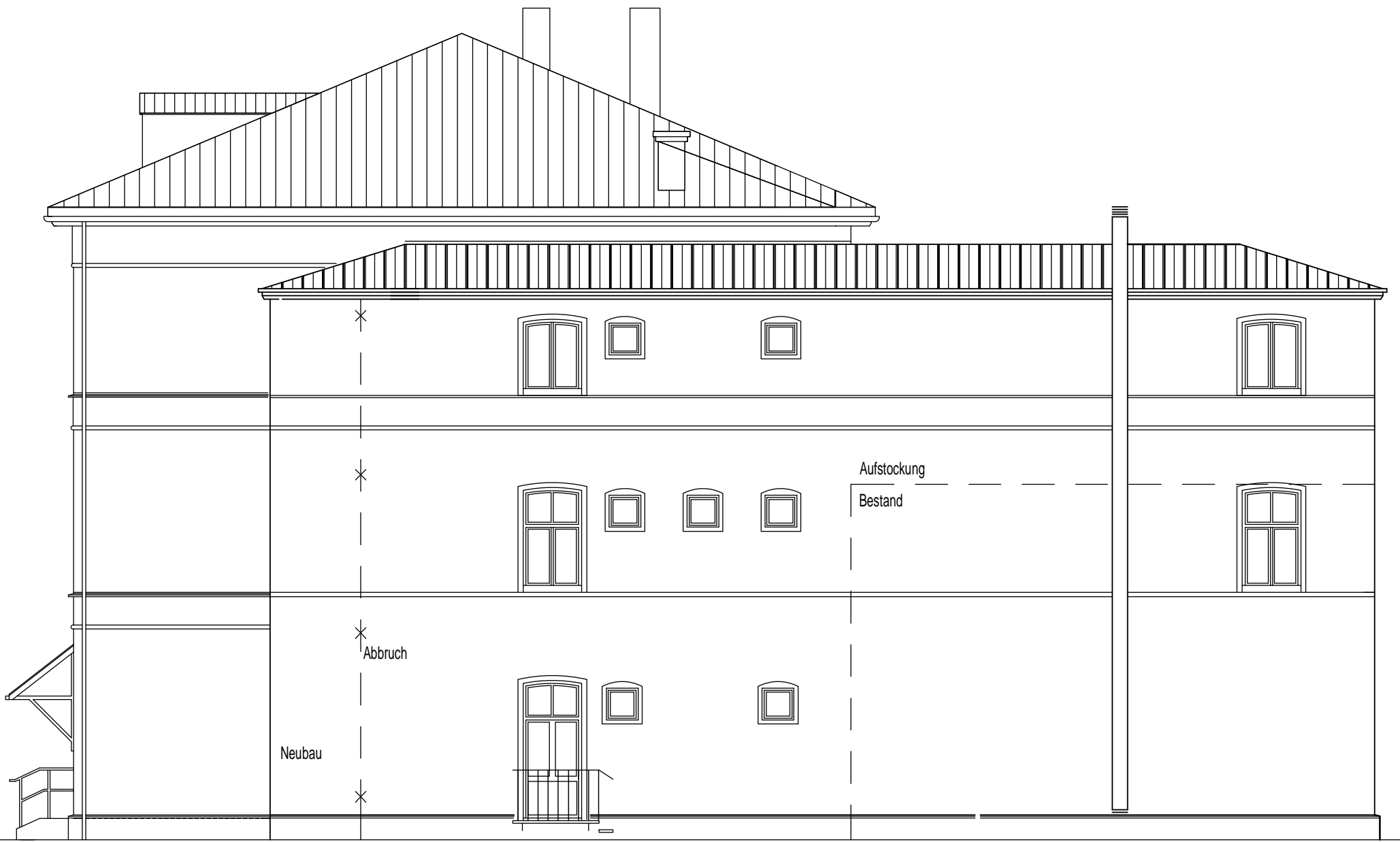
Ansicht Nord - Umbau 2015/03 26.03.2015
